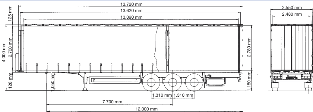
S.CS 24/L – 13.62 EB – Dreiachs-Sattelanhängler mit Curtainsider-Spannplanenaufbau
