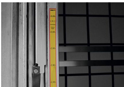
VARIOS-Aufbau: Höhenverstellung in 50 mm-Schritten an der Stirnwand und am Heckportal von 2.800 – 3.000 mm. Ideal für den Wechsel auf Sattelkupplungshöhen für maximale Flexibilität im Transportalltag.
