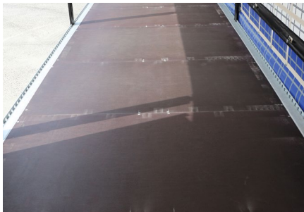
Geklebter Boden vereint längere Haltbarkeit und optimierte Dichtheit. Er ist speziell für hochfrequente Staplerachslasten von 7,5 t konzipiert.
