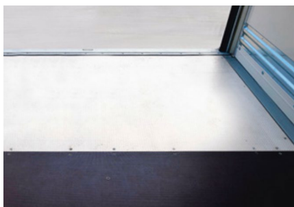
Langlebiger und robuster Siebdruckboden: Bodenbleche am Heckportal schützen die letzte Bodenplatte vor erhöhtem Verschleiß durch häufige Beladung mit einem Gabelstapler und verlängern die Lebensdauer.
