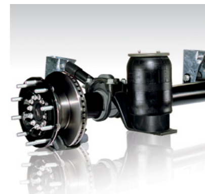
ROTOS-Achse mit zuverlässiger Bremswirkung durch 430 mm Scheiben mit intelligenter Luftkühlung am Achskopf.
