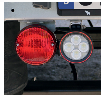
Rückfahrcheinwerfer in LED-Ausführung mit hoher Lebensdauer, am Heck des Chassis befestigt.
