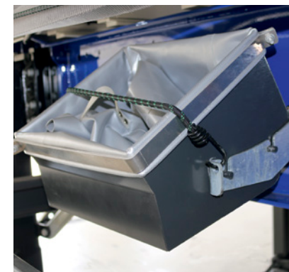
Getreideauslaufrichter für Getreideschieber mit praktischer Parkposition am Chassis oder geschützt im Staukasten.
