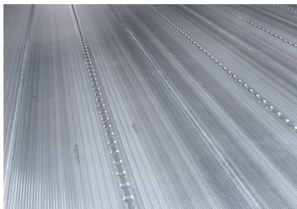
Airline-Boden* mit optimierter Rutschfestigkeit und Lochleiste zur Ladungssicherung: Die verschweißte Bodenwanne erfüllt die Hygienevorschriften, ist schnell zu reinigen und spart Zeit.
