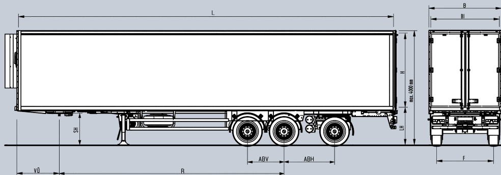
S.KO - 24/LZG Dreiachs - Sattelaufleger - zwangsgelenkt
