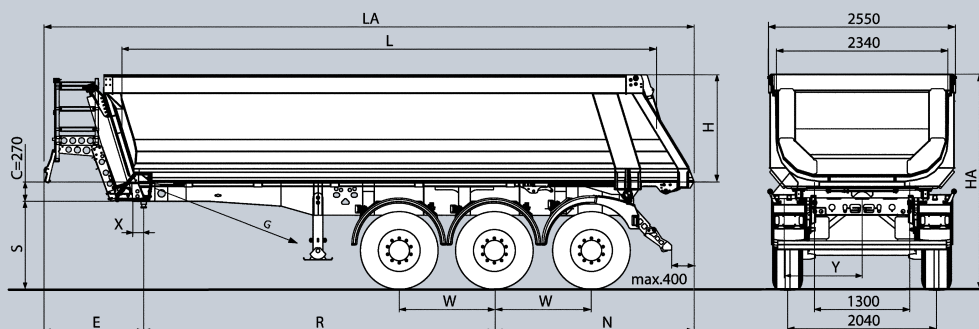
S.KI 24 / 7.2 SL06 SR Semirremolque basculante trasero de tres ejes, con caja de acero y fondo semirredondo
