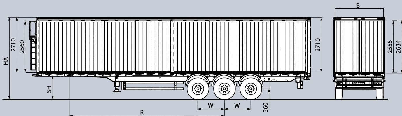
Semirremolque de tres ejes con piso móvil
