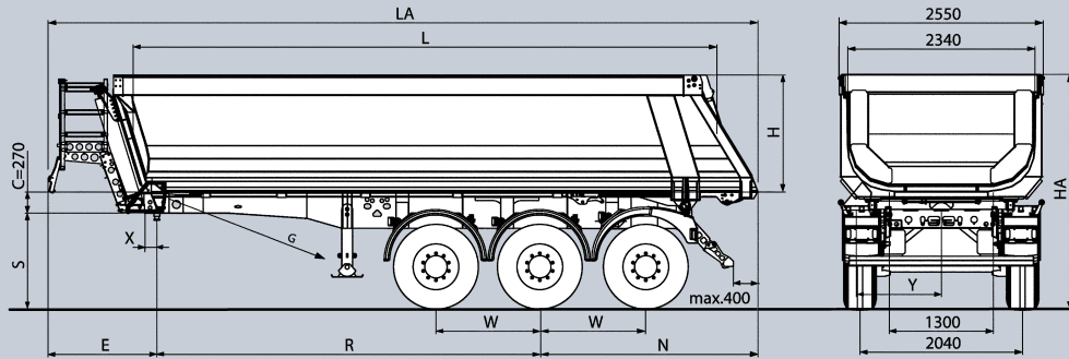
S.KI 24 / 7.2 SL06 SR Semirimorchio a tre assi a ribaltamento posteriore con cassone a sezione circolare in acciaio
