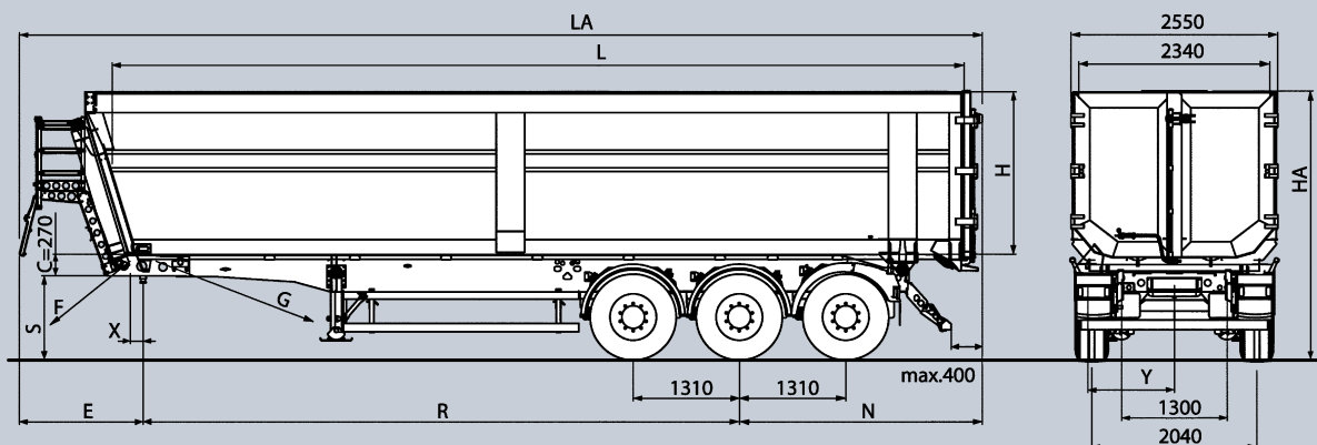
S.KI 24 / 10.5 SL06 SR 3-assige achterlossende kipperoplegger met nde stalen laadbak
