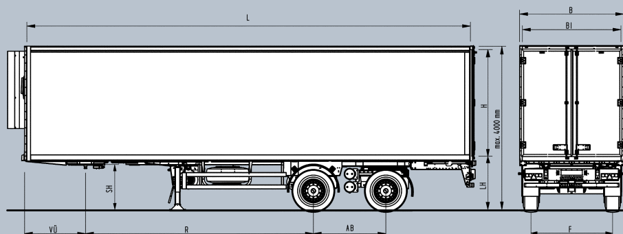
S.KO - 18/LZG Двухосный седельный полуприцеп с принудительно управляемой осью
