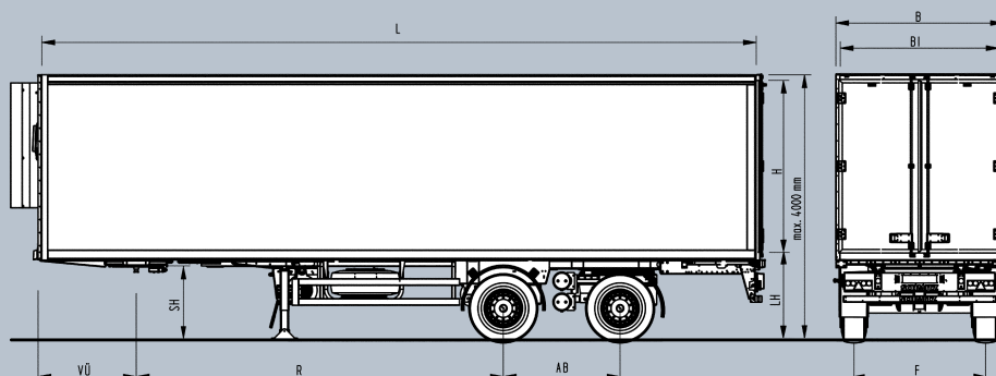
S.KO - 20/LZG Двухосный седельный полуприцеп с принудительно управляемой осью
