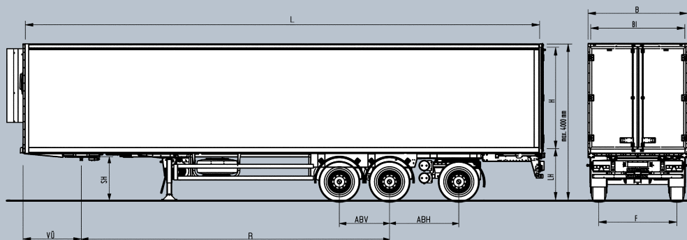
S.KO - 24/LZG Трехосный седельный полуприцеп с принудительно управляемой осью
